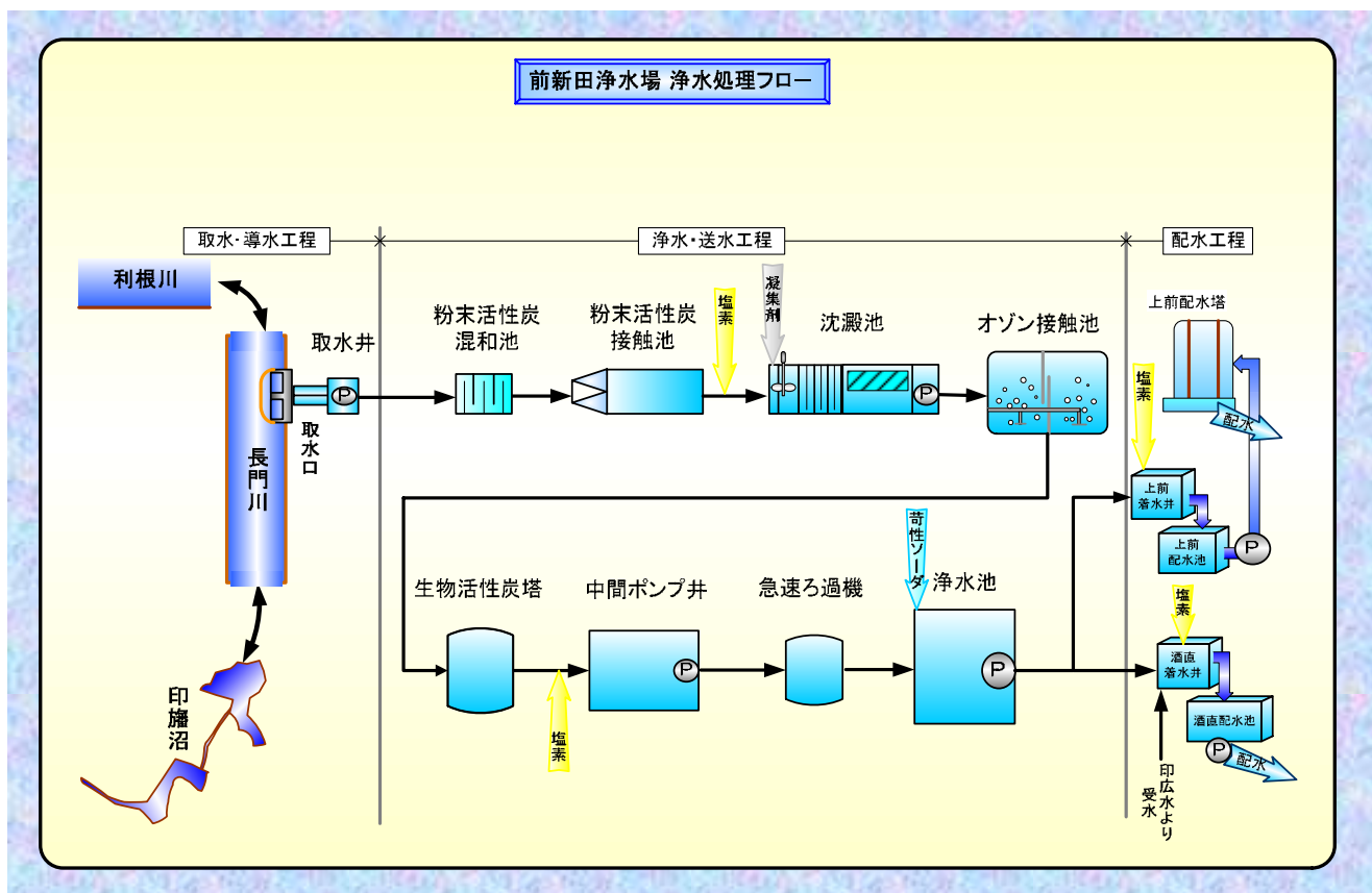
【図 - 2】前新田浄水場 浄水処理フロー
